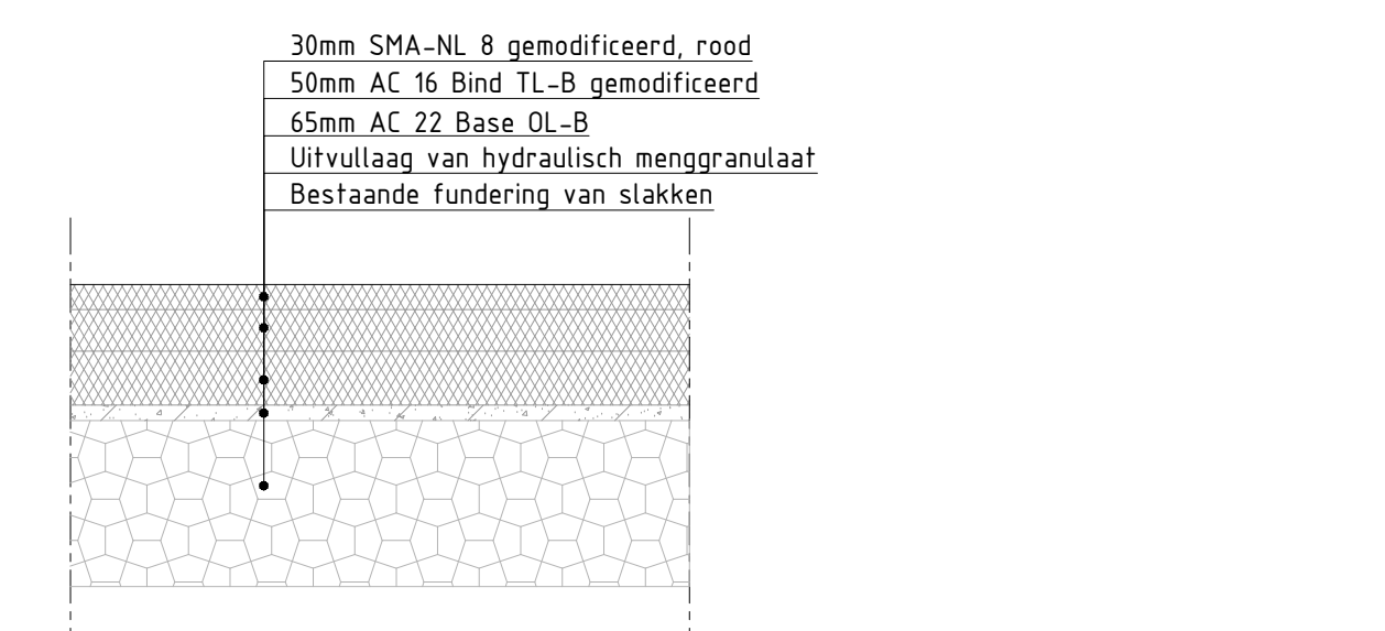
Verhardingsconstructie 10c (f.p.v. fietspad) Schaal 1:10
